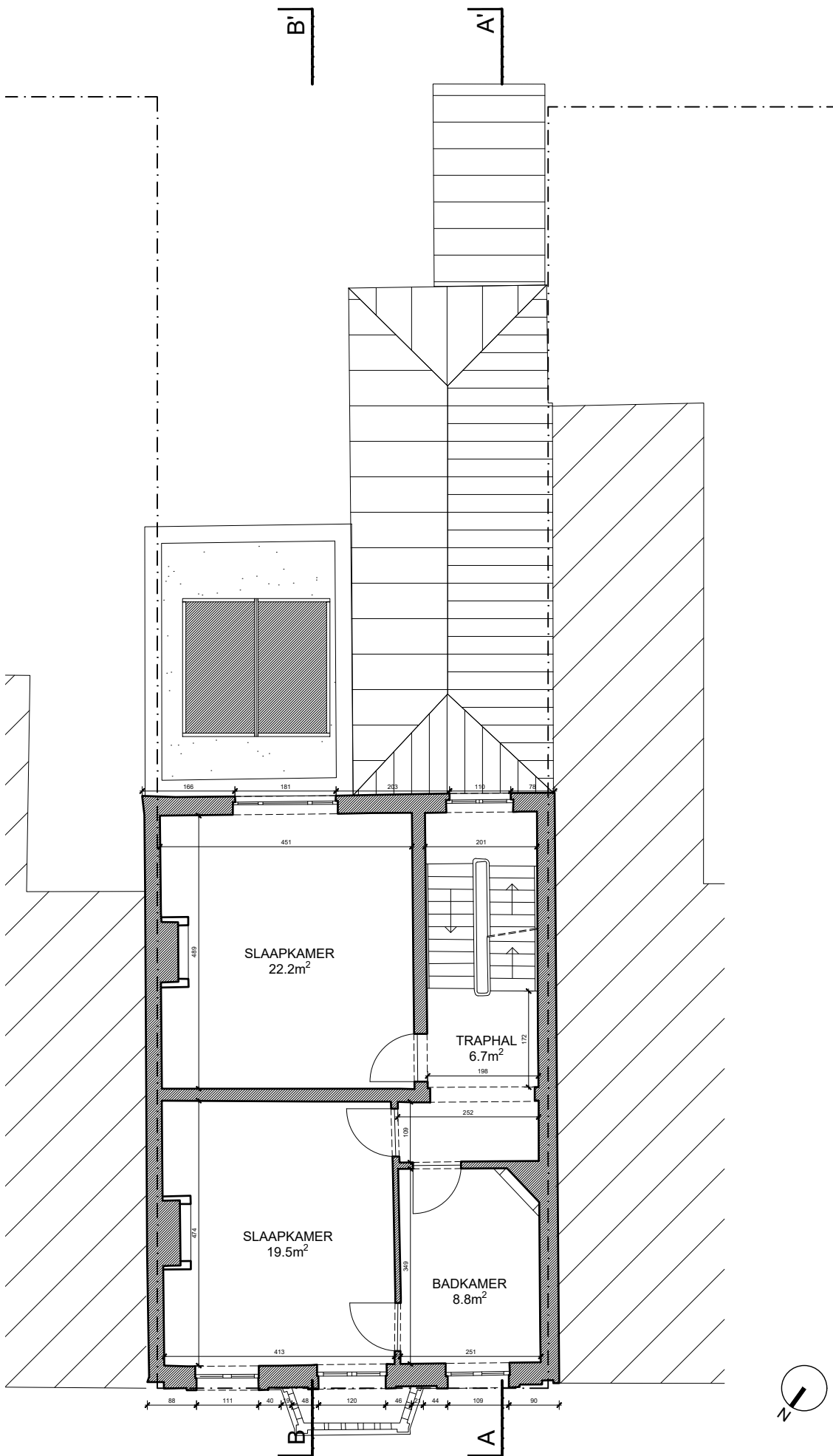
GRONDPLAN NIVEAU +2 BESTAANDE TOESTAND
