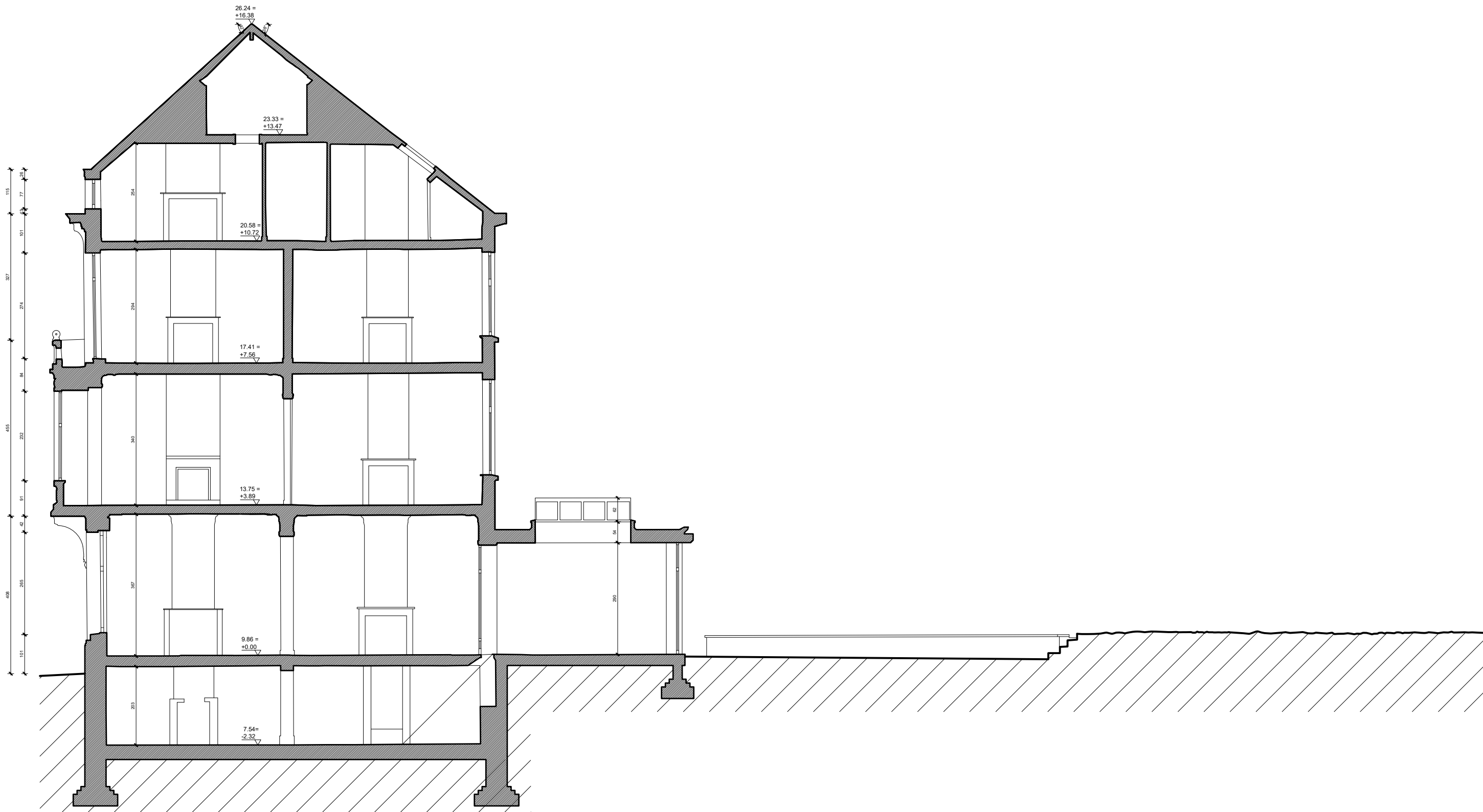
SNEDE SNEDE BB' BESTAANDE TOESTAND
