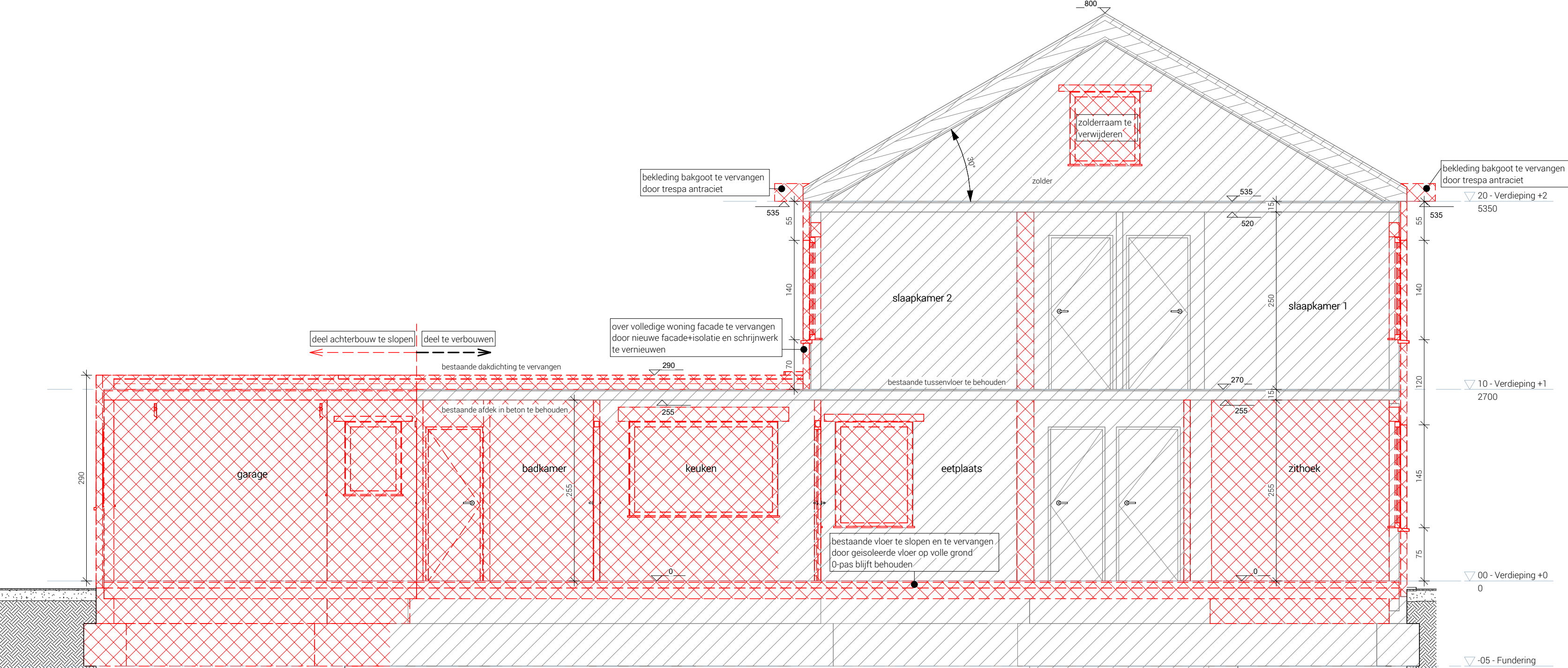
Schaal 1:50 Doorsnede 1 bestaande toestand
