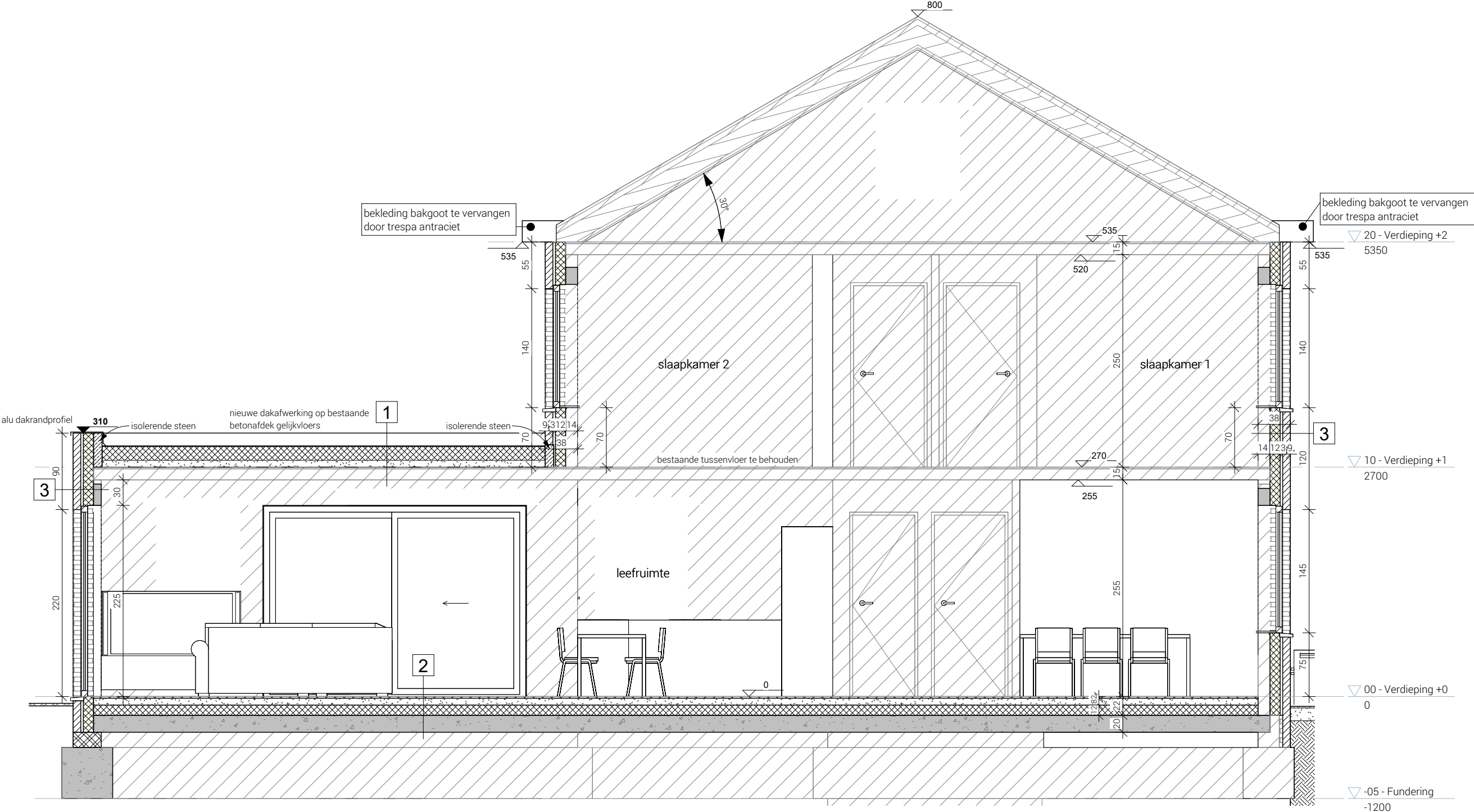
Schaal 1:50 Doorsnede 1 nieuwe toestand
