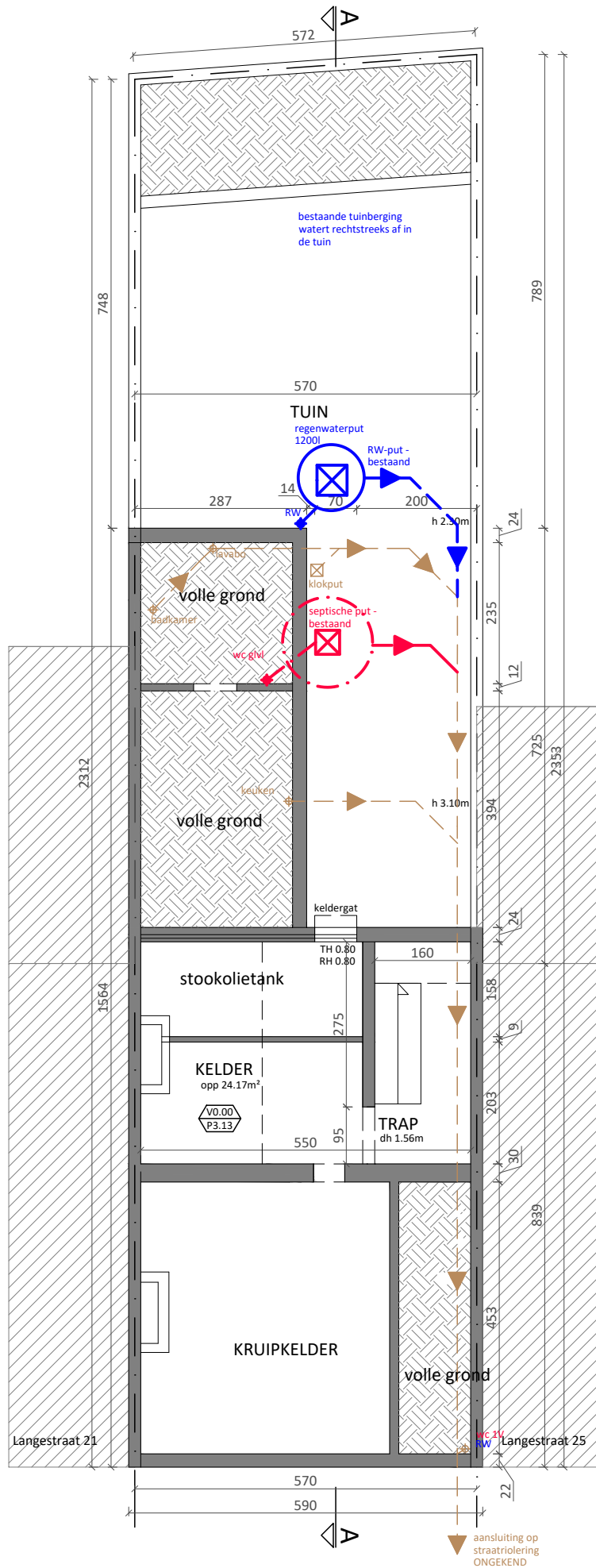
BESTAANDE TOESTAND KELDER FUNDERINGS- en RIOLERINGSSCHEMA ONGEKEND 1-100
