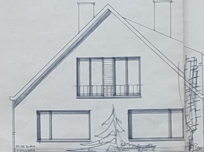
VOORGEVEL
