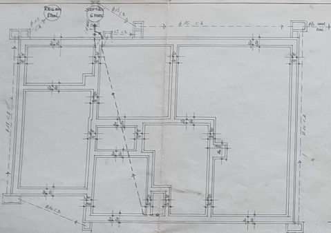
FUNDERINGS-EN ROOIERINGSPLAN.
