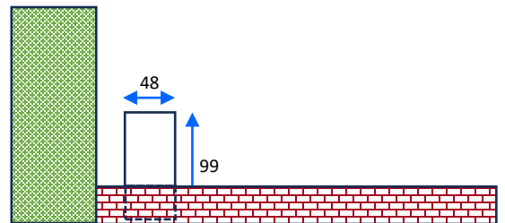
Zijaanzicht links buitenunit
