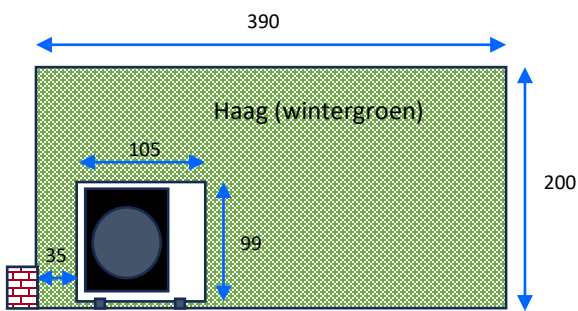
Vooranzicht buitenunit
