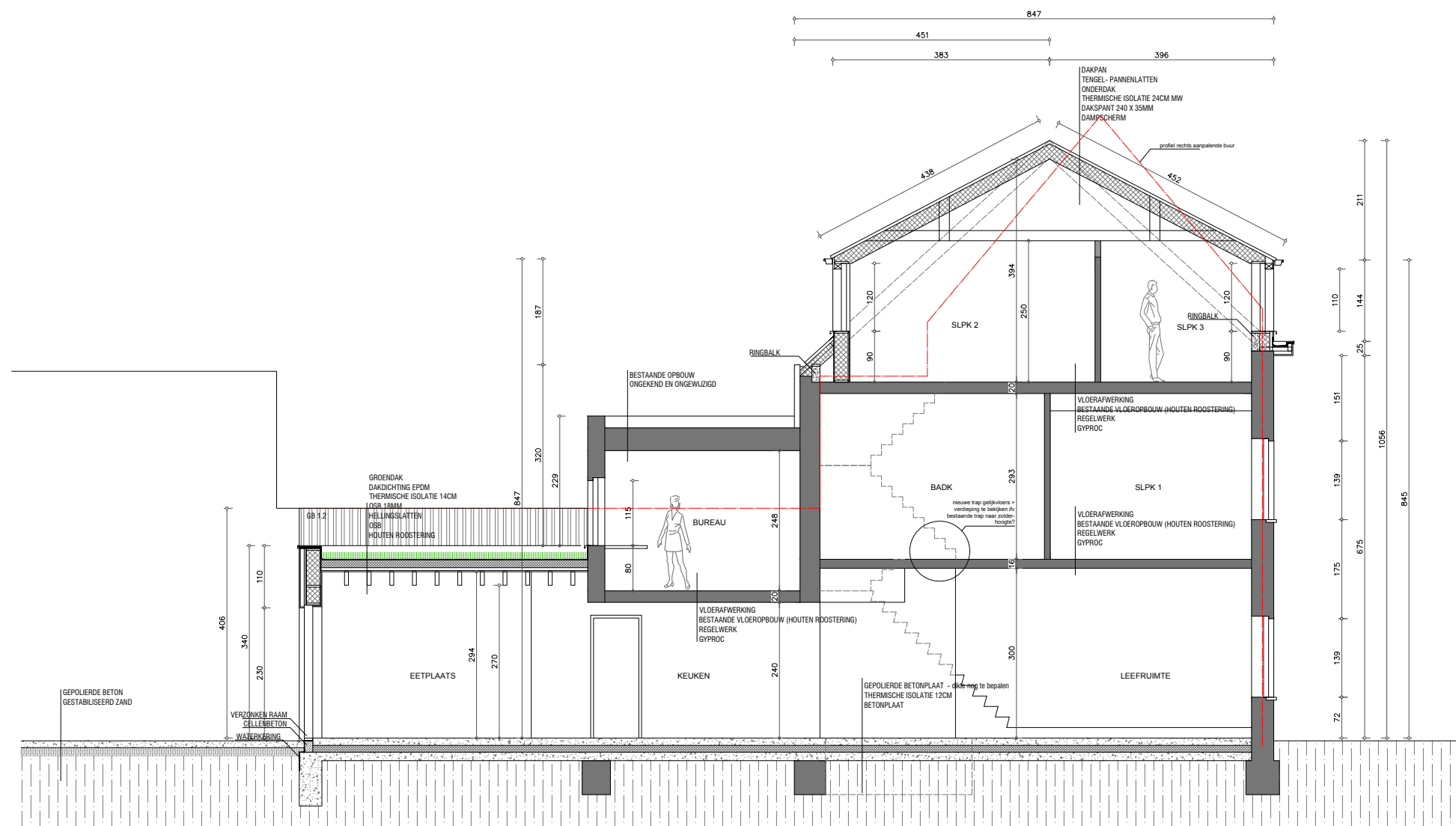
0 2,5m DOORSNEDE A
