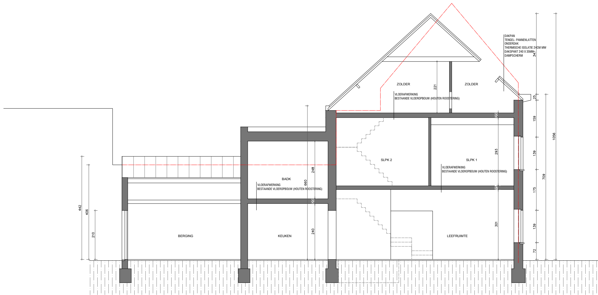
0 2,5m DOORSNEDE A
