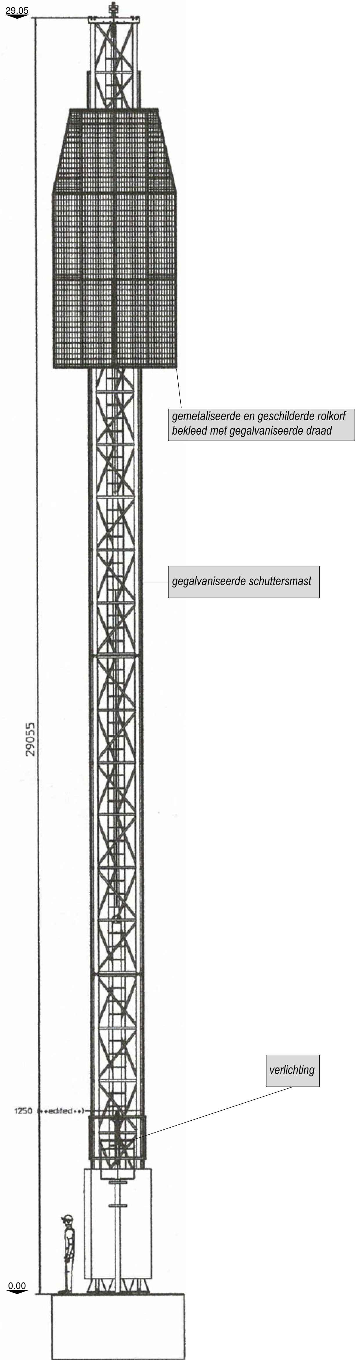
VOORAANZICHT BESTAANDE TOESTAND
