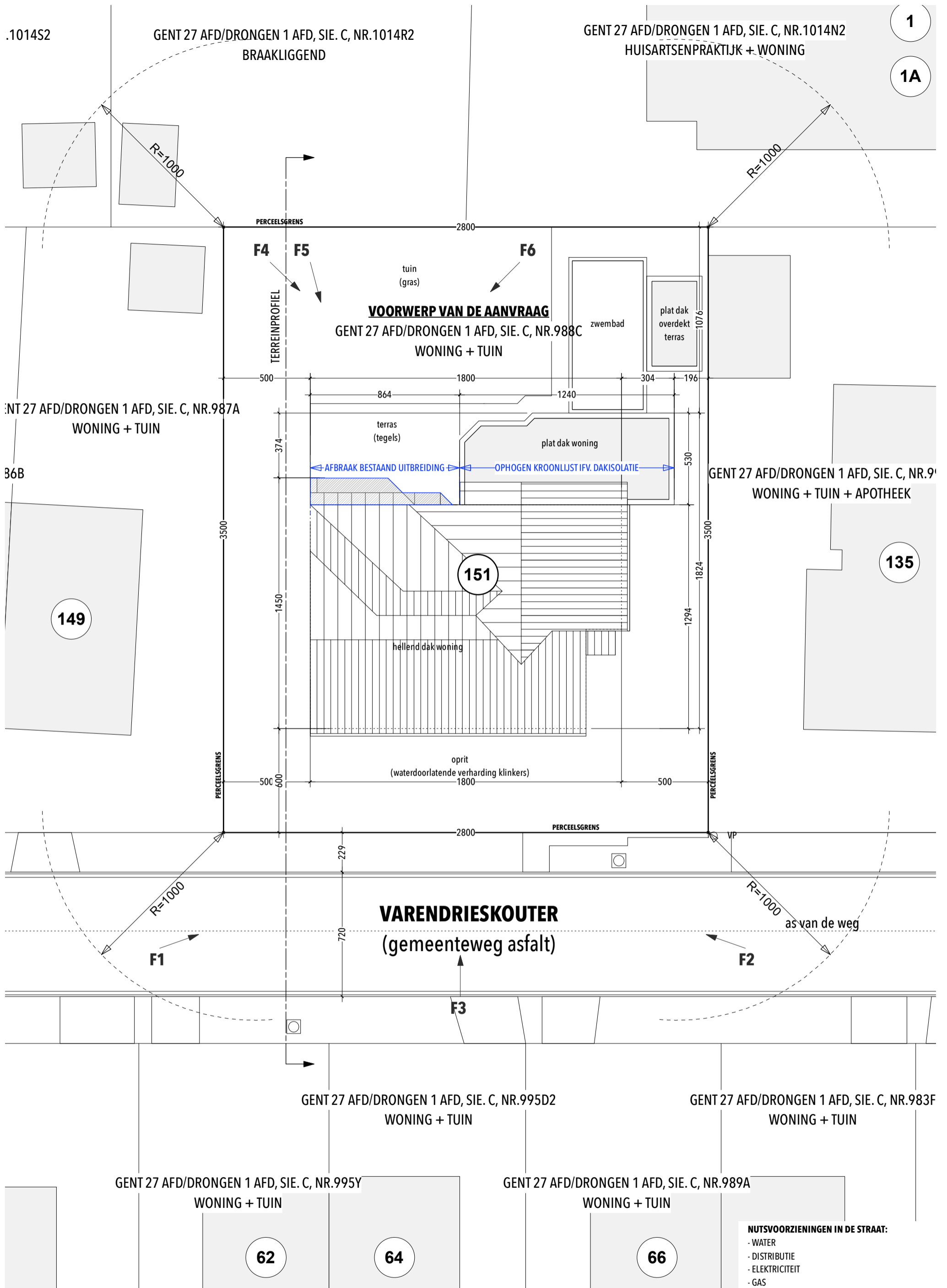
INPLANTINGSPLAN BESTAANDE TOESTAND/AFBRAAK - SCHAAL 1/200
