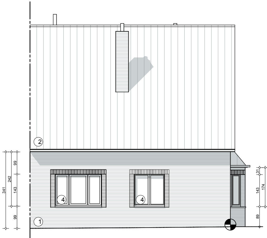
Gevel Serafien Van Cauwenbergelaan Bestaande toestand
