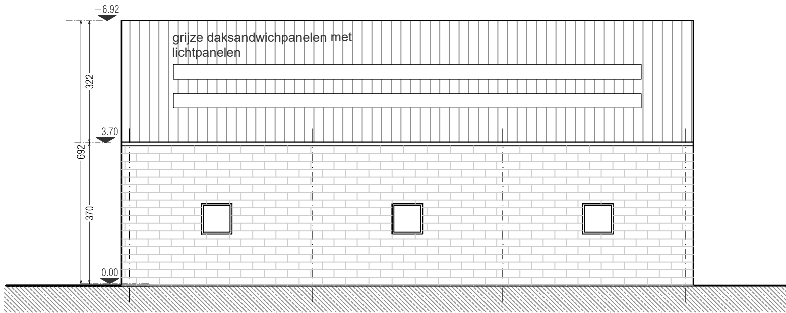
ZIJAANZICHT RECHTS SCHAAL 1/100
