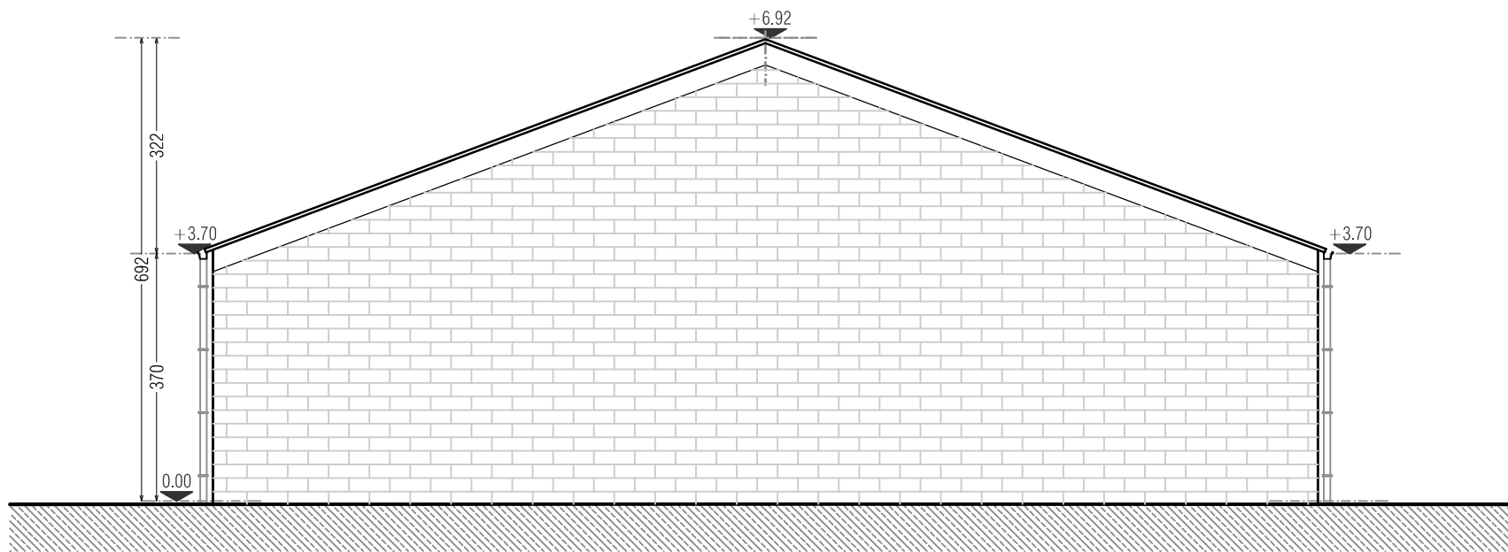
ACHTERAANZICHT SCHAAL 1/100
