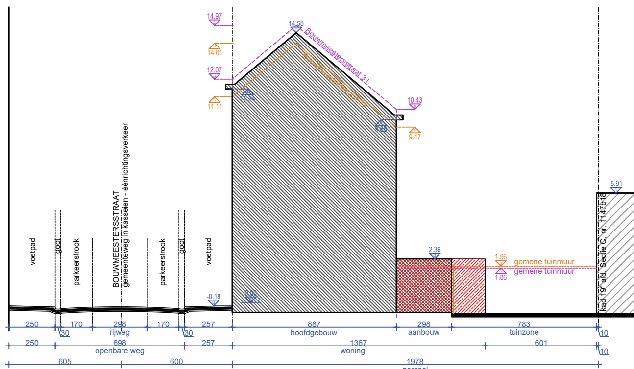
TERREINPROFIEL bestaande toestand - 1/200
