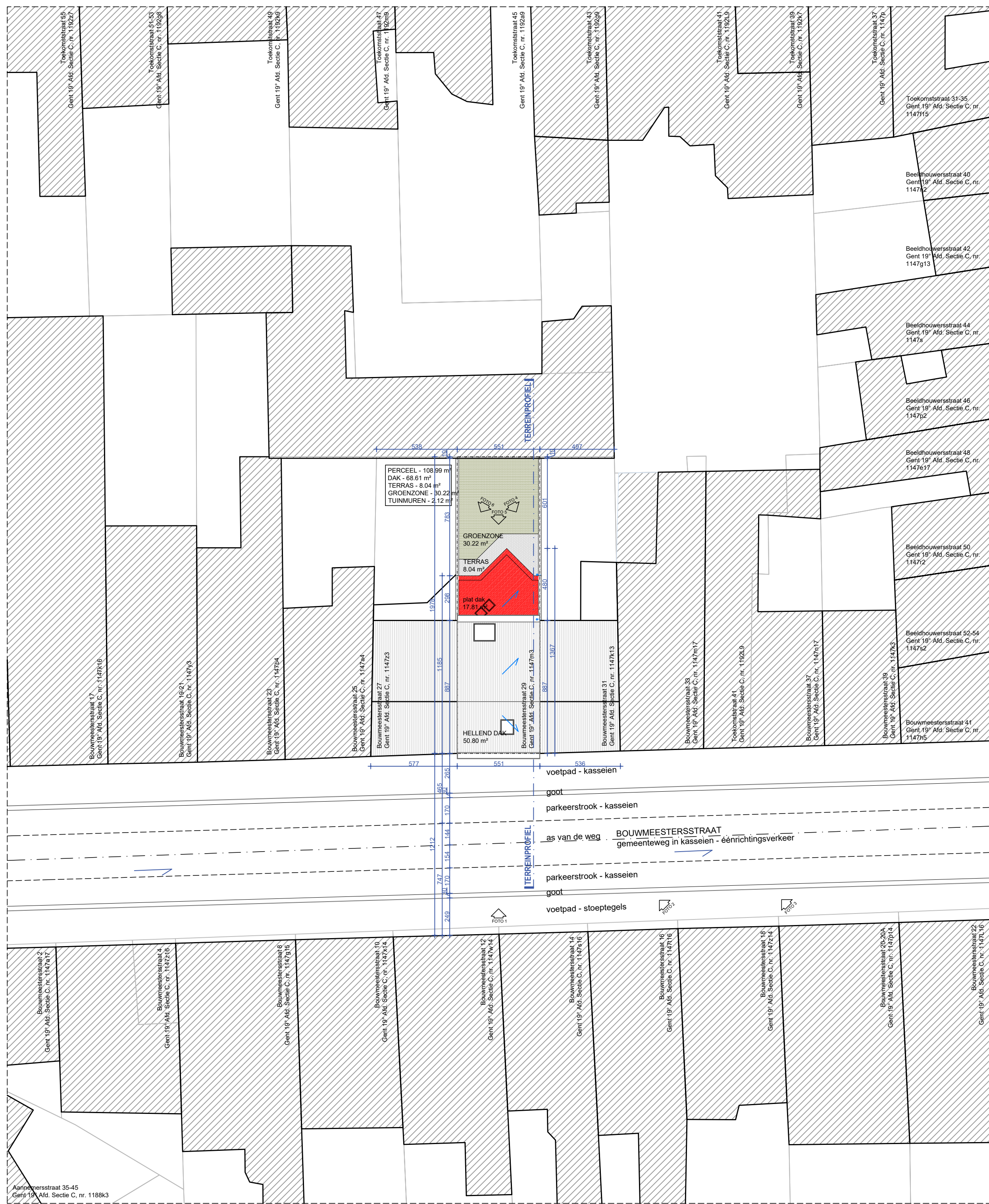
INPLANTINGSPLAN bestaande toestand - 1/200
