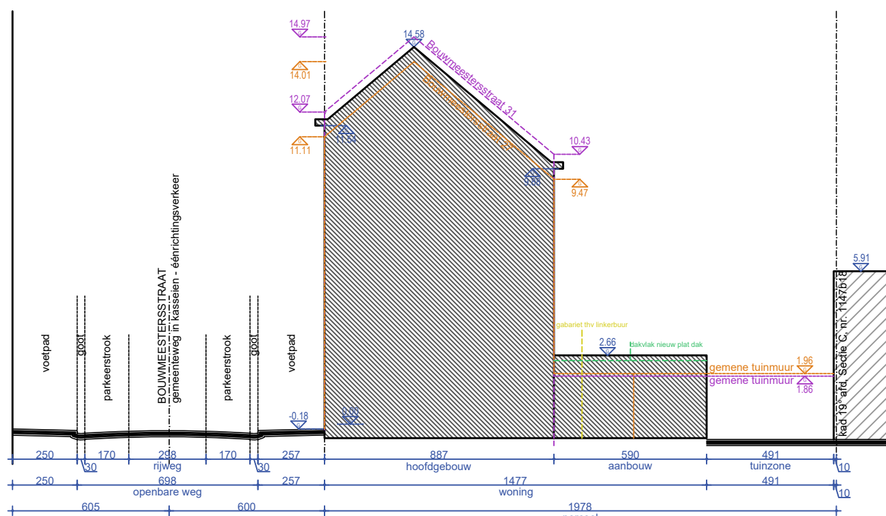
TERREINPROFIEL nieuwe toestand - 1/200
