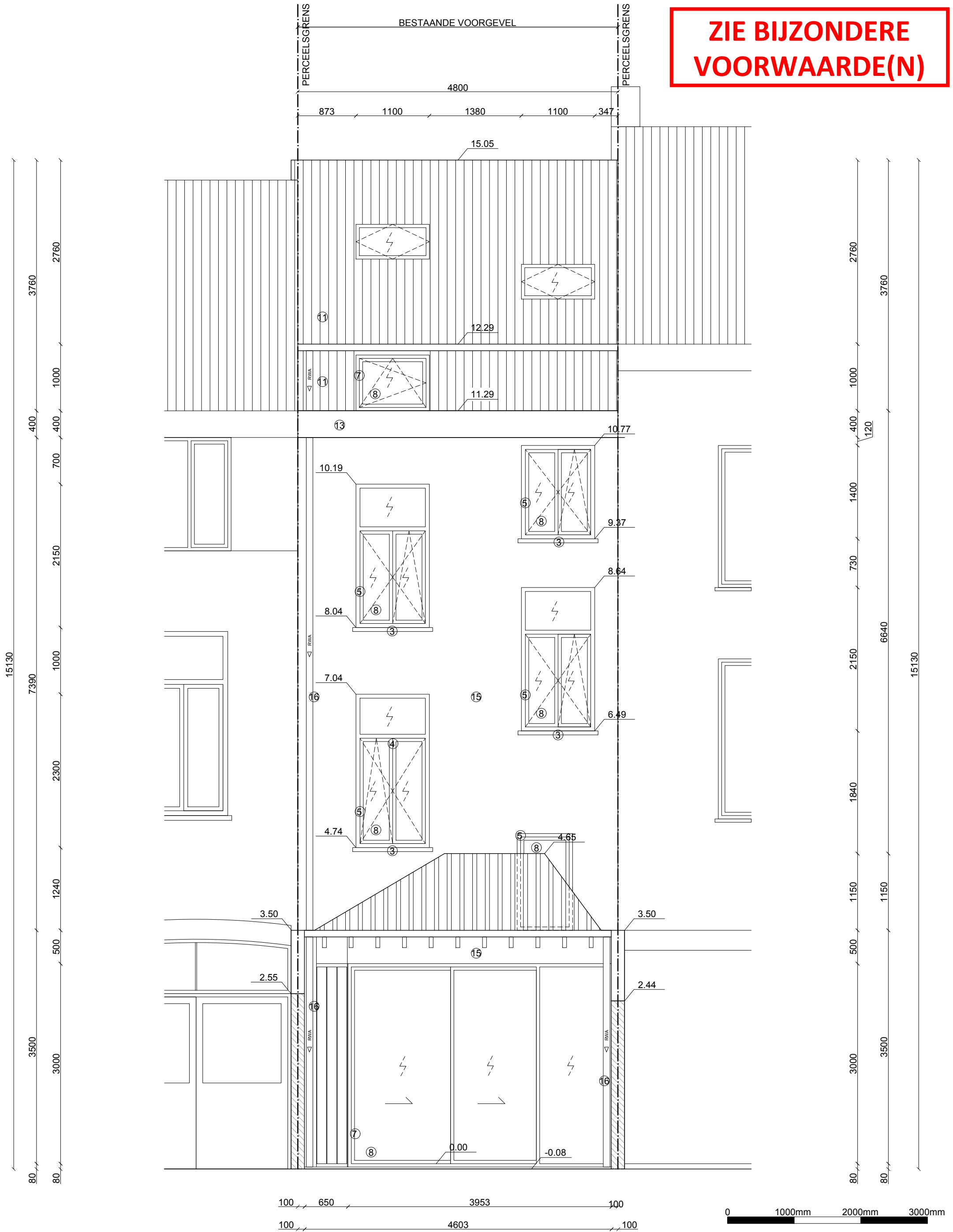
G_N_ACHTERGEVEL
