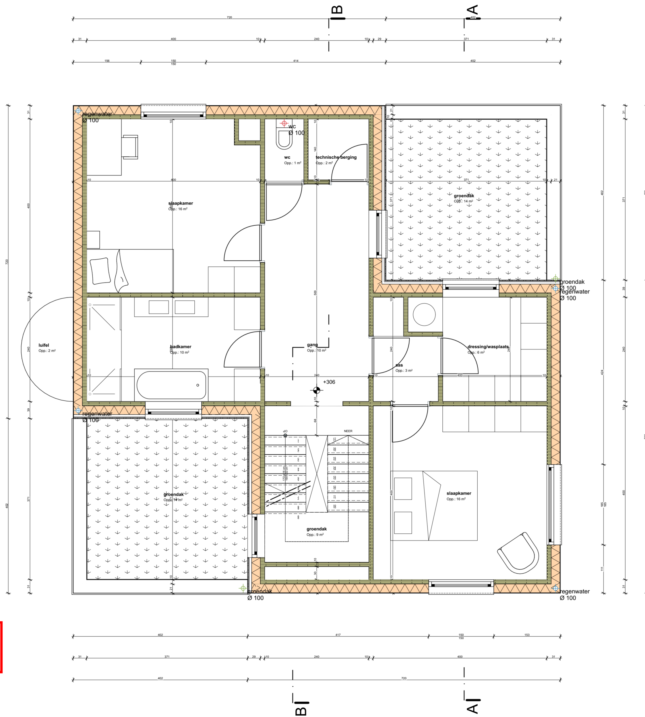
01_verdieping - 1:50
