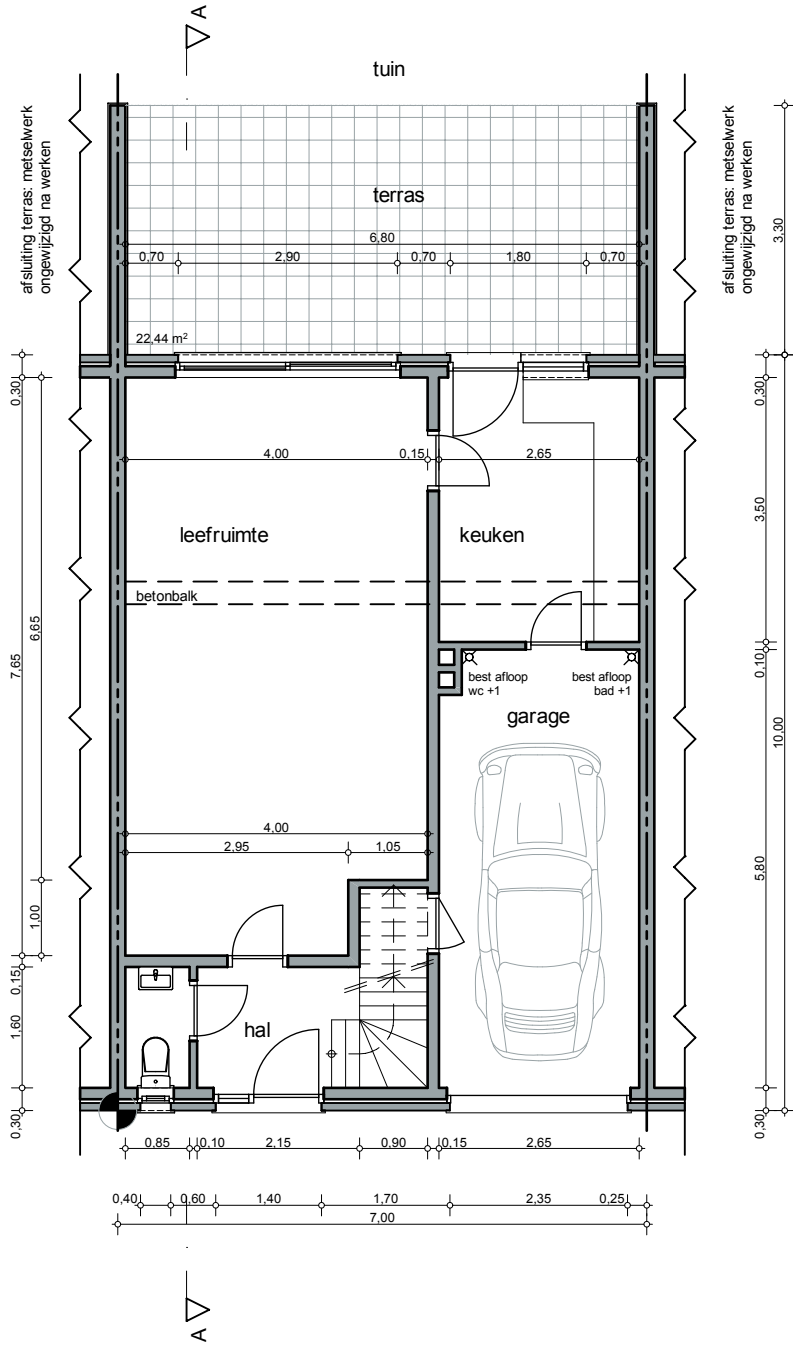
Grondplan gelijkvloers Bestaande toestand - schema - ongewijzigd na de werken
