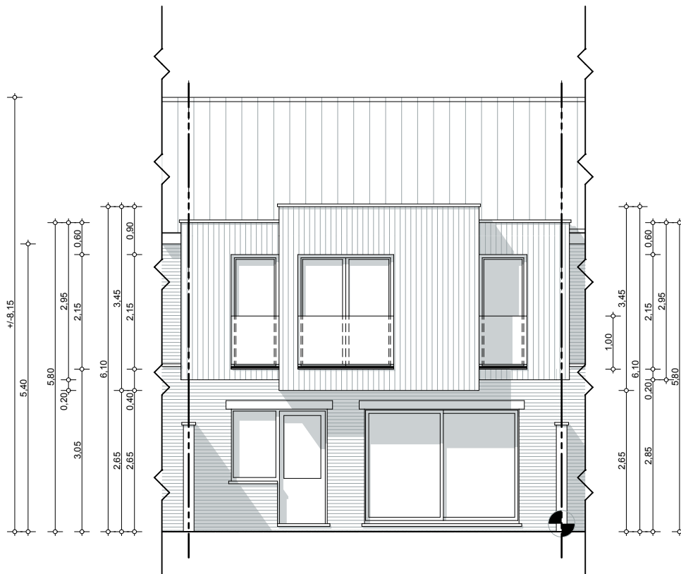
Gevelaanzicht achtergevel Nieuwe toestand (met uitbreiding op verdieping)
