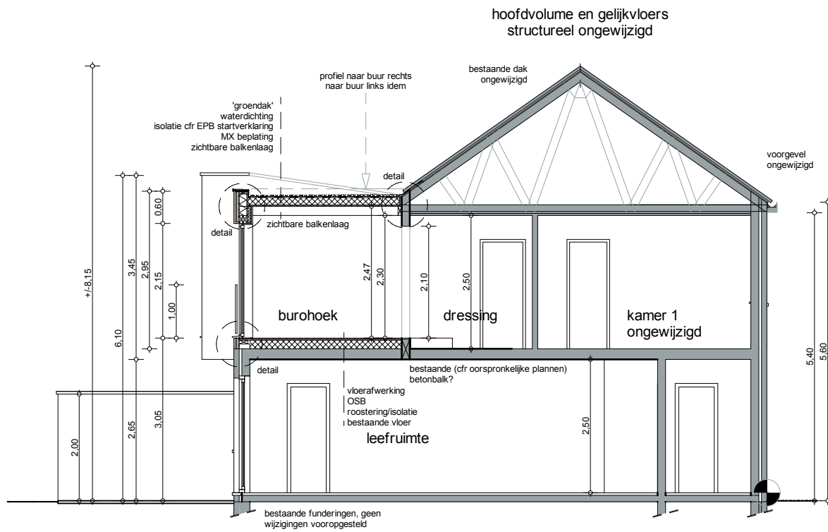
Principeddoorsnede - schema Nieuwe toestand (met uitbreiding op verdieping achteraan)
