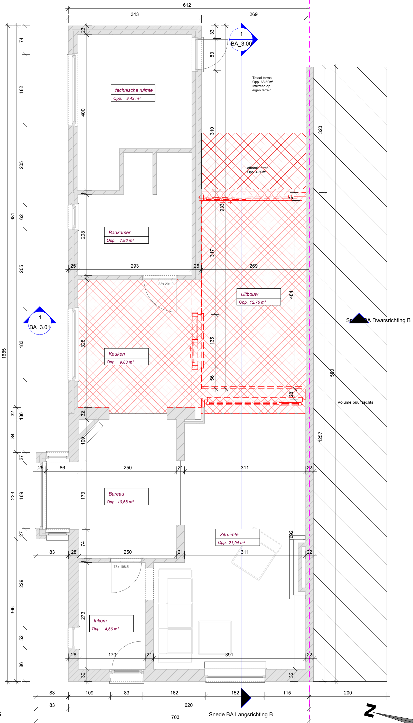
BA_1.00 P_B_1.00_Grondplan Gelijkvloers
